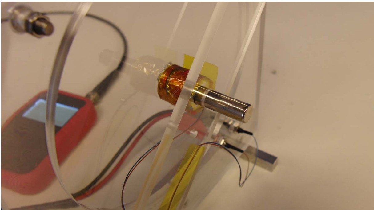
Plexiglasmikrofon von hinten (Spule auf OHP-Folie und feststehender Magnet) Das Ende des Magneten ist in der Spulenmitte. (Die Folie ist zwischen zwei Plexiglasplatten mit Öffnung eingeklemmt.)
